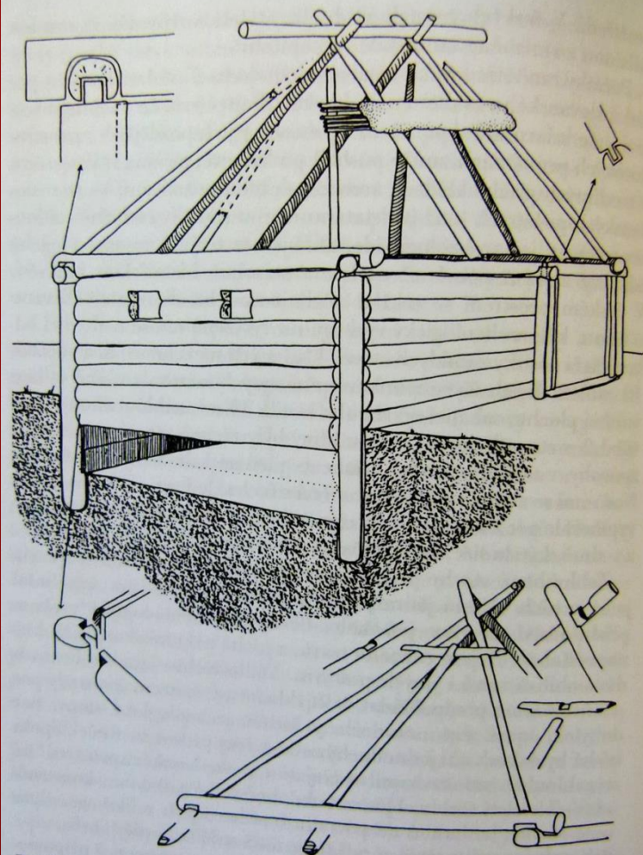
Raně středověká částečně zahloubená stavba rekonstruovaná podle archeologického výzkumu v Březně u Loun
